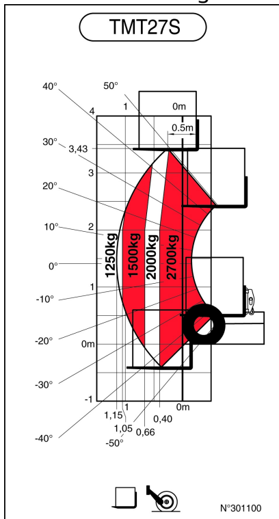
Ábaco de carga
