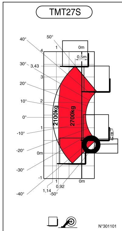
Máquina sobre estabilizadores con horquillas
